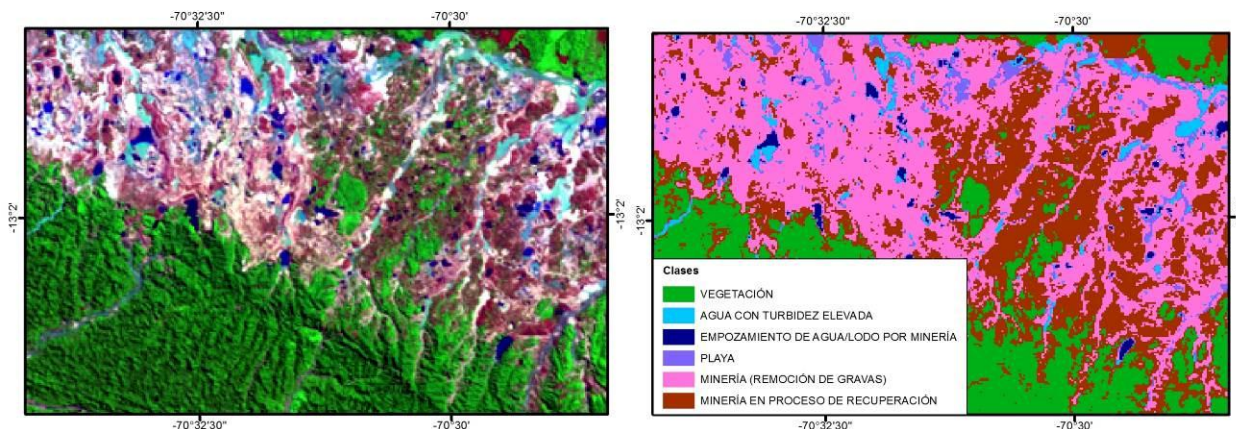
Figura N° 3. Izquierda: Composición LANDSAT RGB: 742 del área de Huepetuhe, (imagen LANDSAT de fecha 23/08/2007); Derecha: Clasificación de la imagen LANDSAT (de fecha 23/08/2007) usando método de clasificación supervisada SAM.
